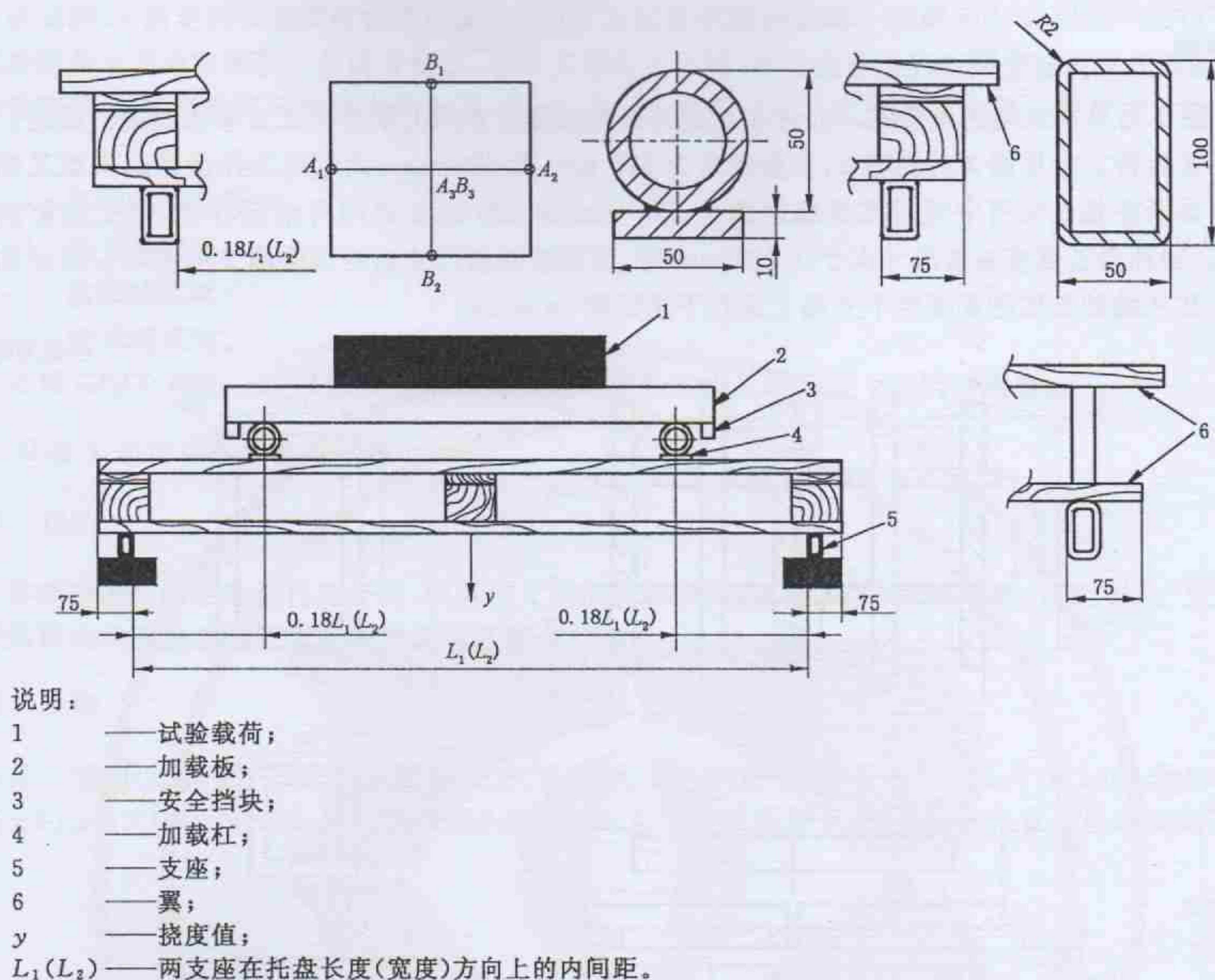
图 1 抗弯试验
