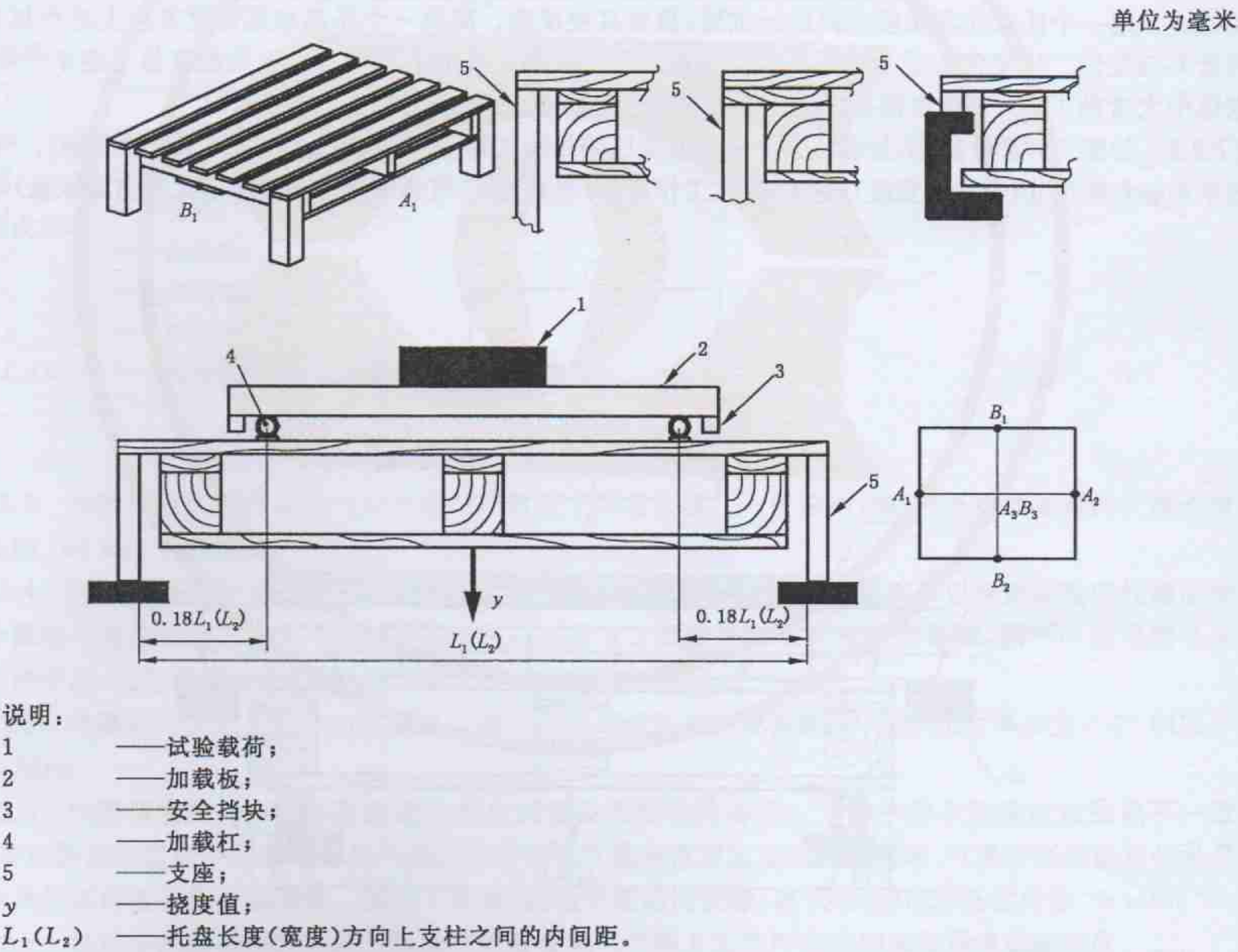
图 6 翼托盘抗弯试验
